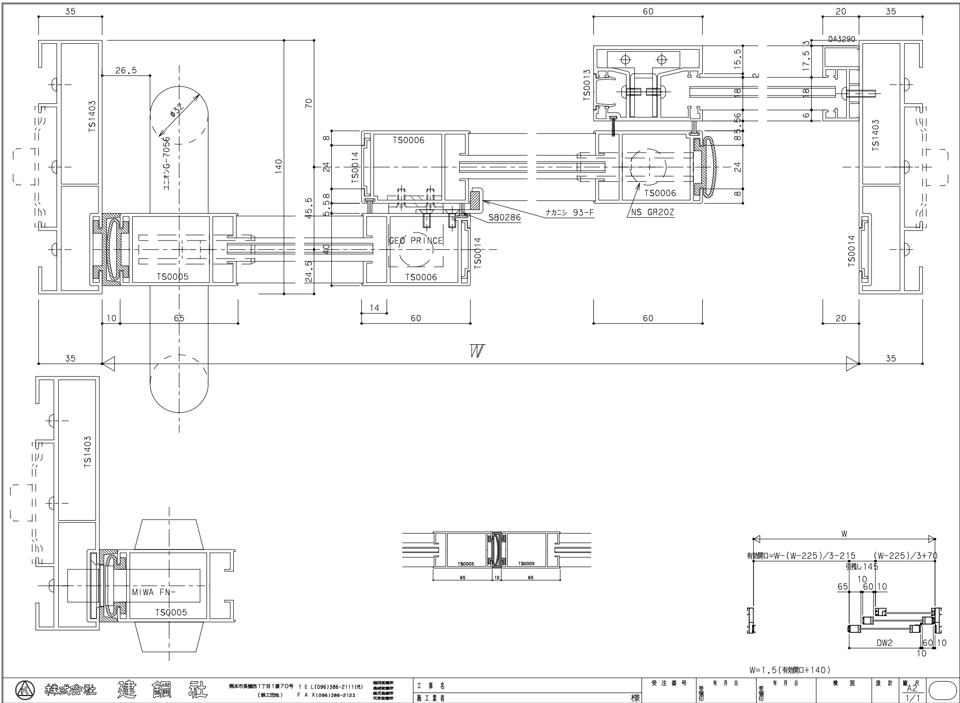
ツインスライダー横断面図ガイドローラー型
