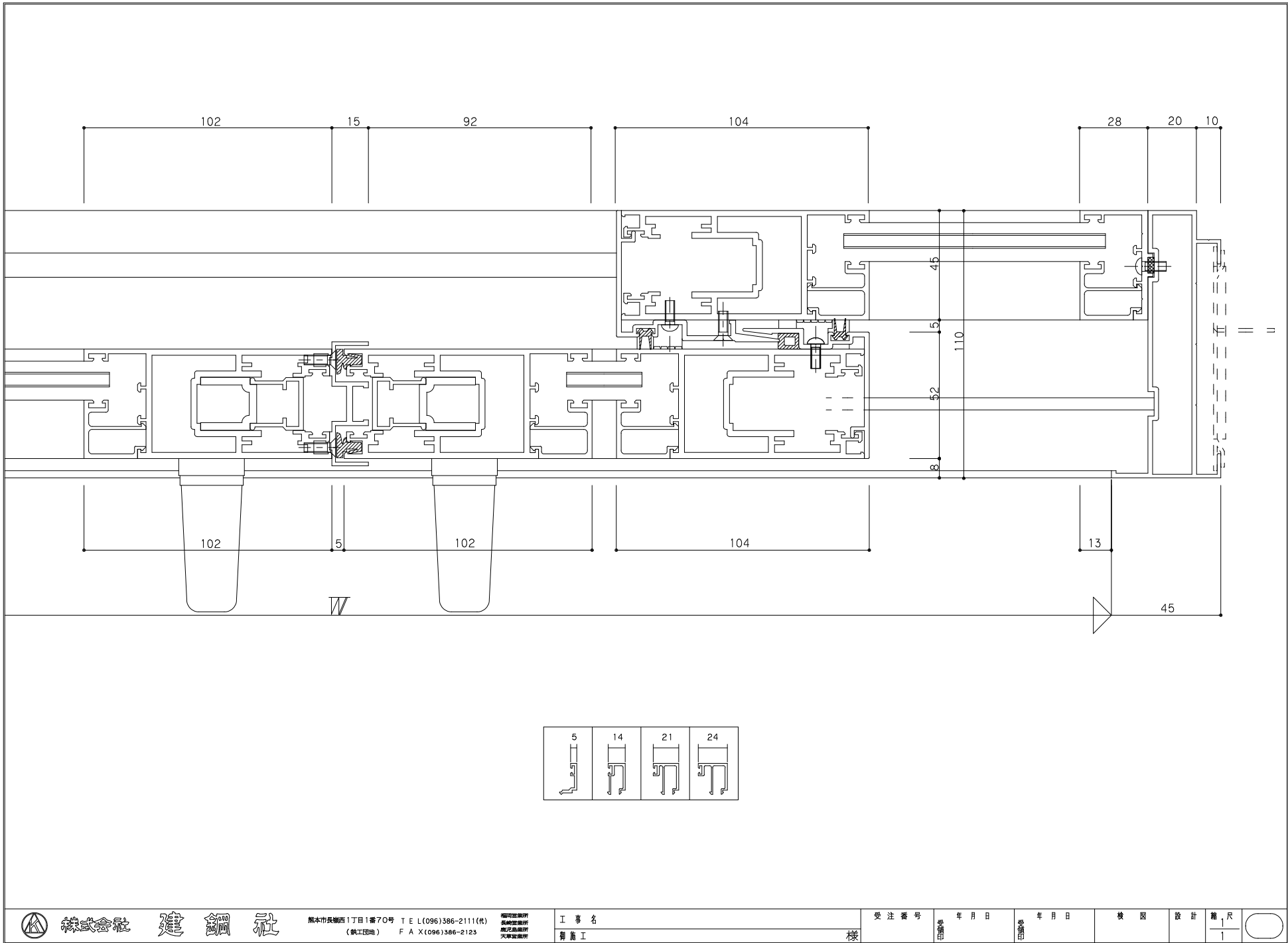
ヘーバントシーバー両引き分け横断面
